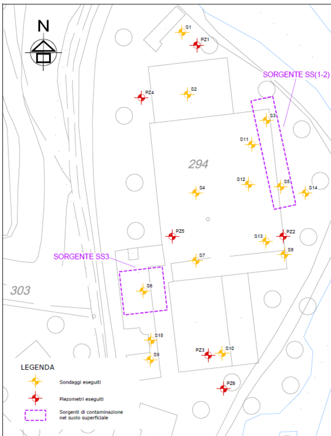
Figura 1 – Planimetria con sorgenti di contaminazione nel suolo superficiale
