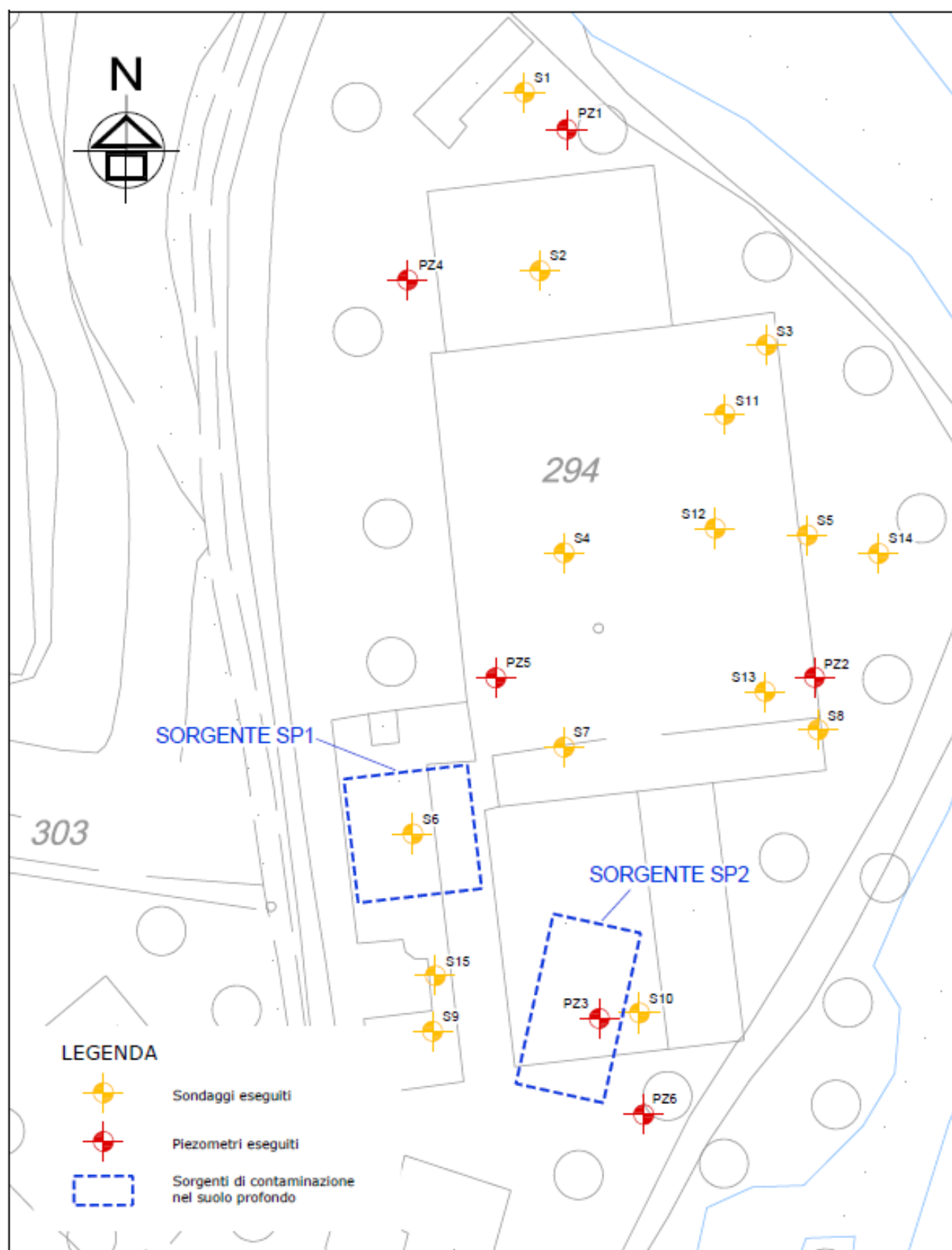
Figura 2 – Planimetria con sorgenti di contaminazione nel suolo profondo
